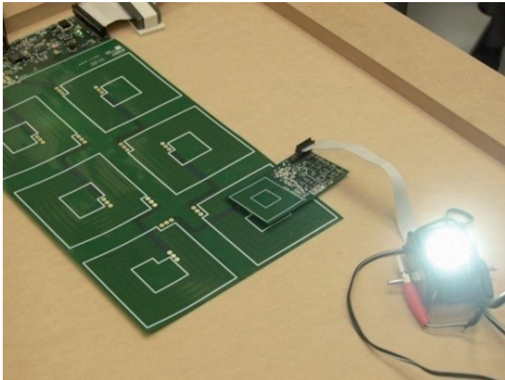
Abbildung 2: Matrix mit mehreren Sendespulen für eine hohe Abdeckung.
