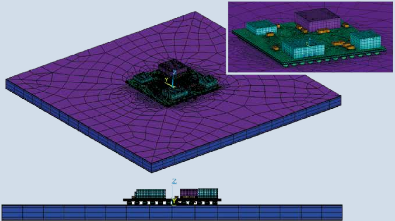
Finite-Element-Modell des USeP-Moduls mit Sensorbestückung.
