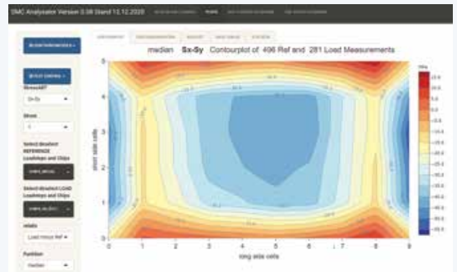
Stresschip-Auswertesoftware (Median Differenzstress von 50 Chips).
