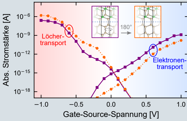
Transferkennlinien von Silizium-basierten rekonfigurierbaren Feldeffekttransistoren mit NiSi 2 -Kontakten. Änderungen in der atomaren Struktur ändern maßgeblich die Symmetrie zwischen Elektron- und Lochströmen.
