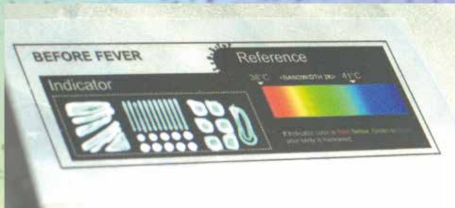
Technologiedemonstrator zur Temperaturindikation bei Fieberpatienten durch Drucken von thermochromen Tinten auf hautverträgliche Substrate.
