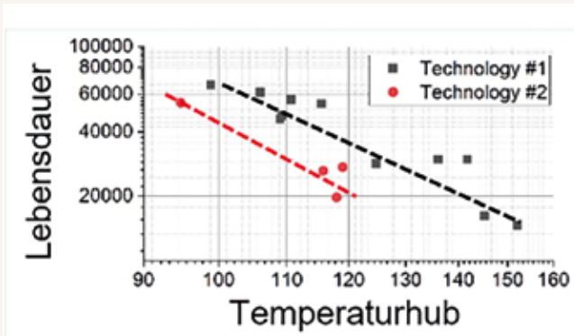
Lebensdauercurven für verschiedene, im Projekt CosmoDU untersuchte Leistungsmodul-Aufbauvarianten.
