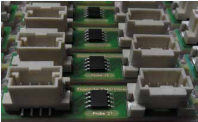
Auf Testleiterplatten gelötete Stresschip-Packages.
